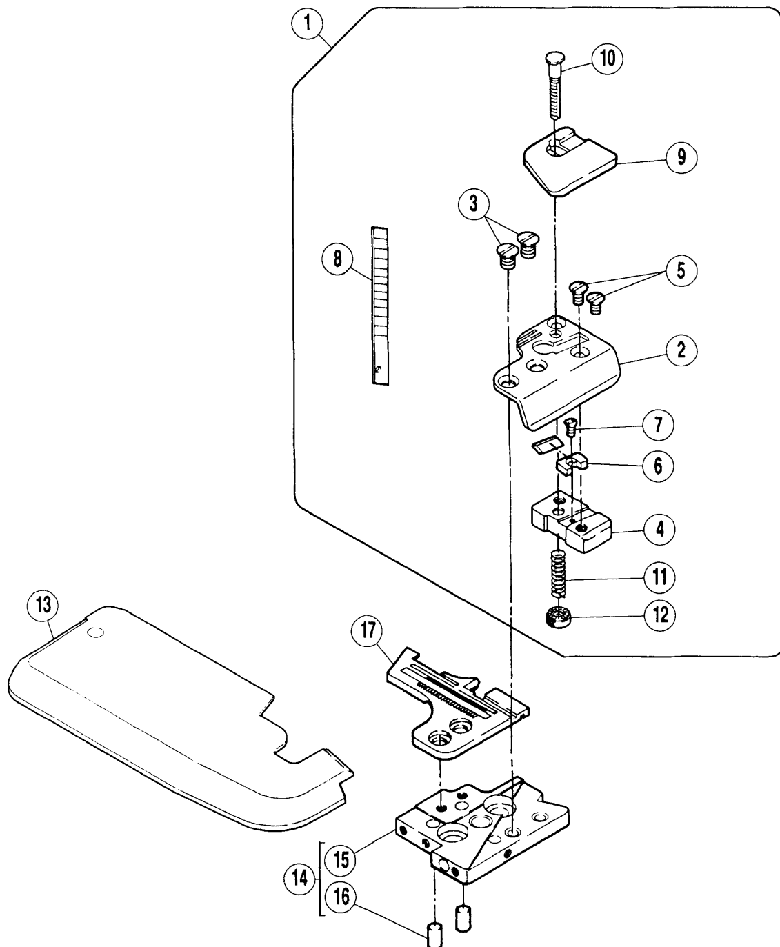
M652 ゲージパーツ表
